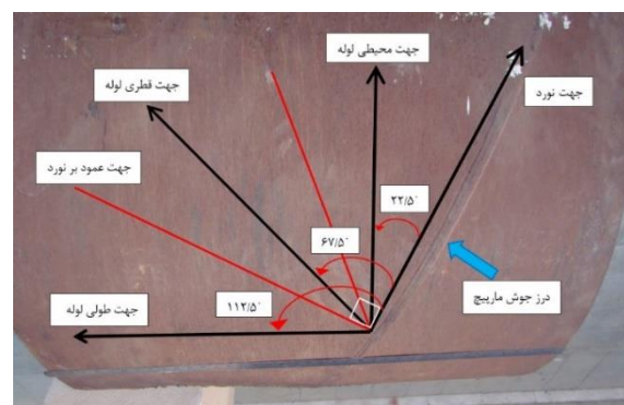
شکل ۱) تصویر کلی از لوله به‌همراه زوایای متناظر جهت‌های اصلی لوله با زوایای نمونه نسبت به جهت نورد.
