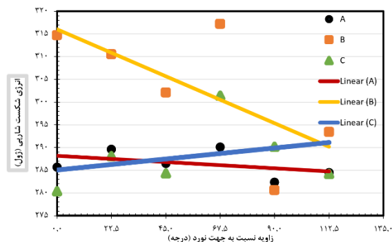
شکل ۹) نمودار تغییرات میانگین انرژی شکست شاری نمونه‌های با هر سه جهت شیار متفاوت A، B و C برحسب زاویه نسبت به جهت نورد
