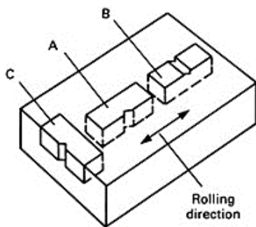
شکل ۲) موقعیت و جهت‌گیری‌های نمونه‌های شاری با جهت شیار A, B و C در زاویه صفر درجه نسبت به جهت نورد در فلز پایه.
