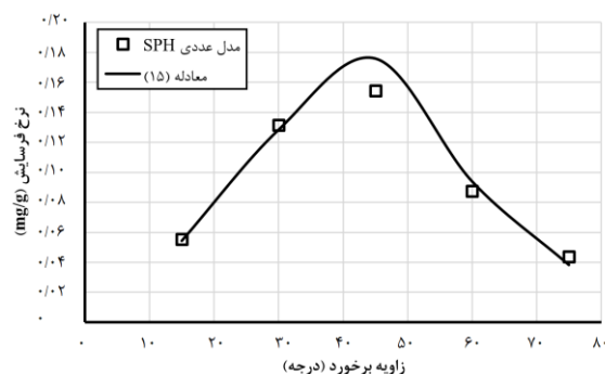
شکل ۸ مقایسه نتایج حاصل از مدل عددی SPH و مدل پیش‌بینی از معادله (۹) در سرعت ۴۵ متر بر ثانیه
