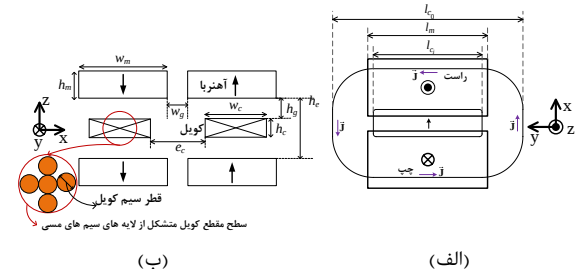
شکل (۲) پیکربندی و پارامترهای طراحی محرک الکترومغناطیسی: (الف) نمای بالا، (ب) نمای جانبی
