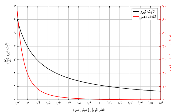
شکل ۵) منحنی ثابت نیرو و اتلاف اهمی بدست آمده از محاسبات تحلیلی در مقابل تغییرات قطر سیم سیم‌پیچ
