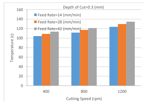
شکل ۳) تأثیر سرعت برشی و نرخ پیشروی بر دمای ماشینکاری با عمق براده ۰/۳ میلی‌متر
