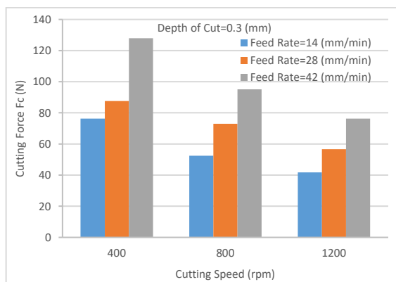
شکل ۲) تأثیر سرعت برشی و نرخ پیشروی بر نیروهای برشی با عمق براده ۰/۳ میلی‌متر
