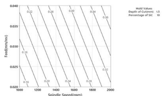
شکل ۷ نمودار اثر برهمکنش نرخ پیشروی و سرعت اسپیندل
