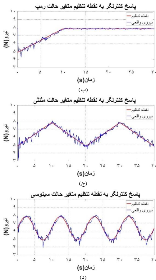
شکل ۲) پاسخ کنترلر PID به (الف) نقطه تنظیم ثابت (ب) نقطه تنظیم متغیر حالت رمپ (ج) نقطه تنظیم متغیر حالت مثلثی (د) نقطه تنظیم متغیر حالت سینوسی
