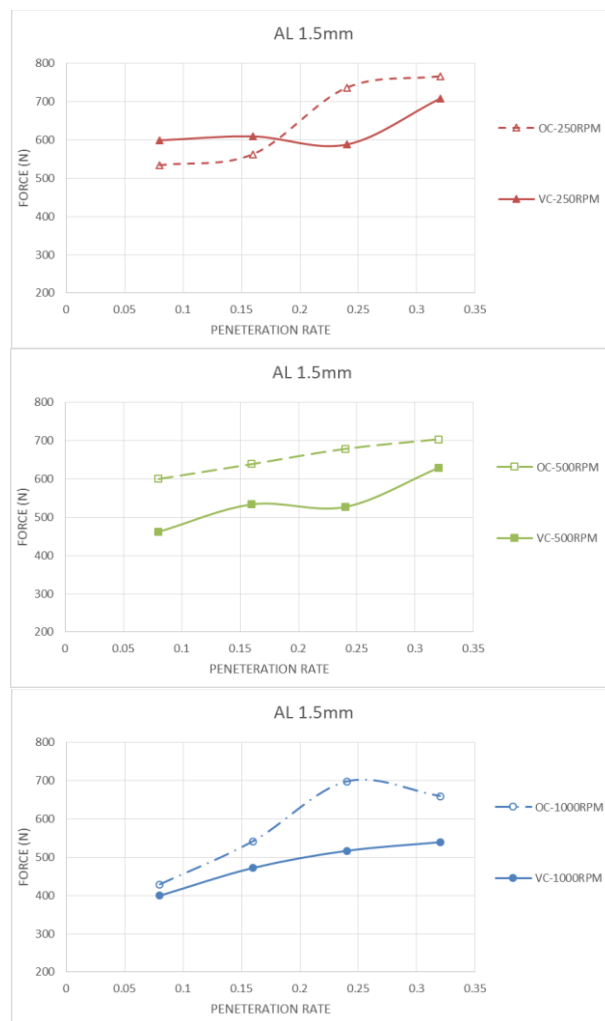
شکل ۷) نیروی محوری سوراخکاری آلومینیوم ۱/۵ میلیمتر
