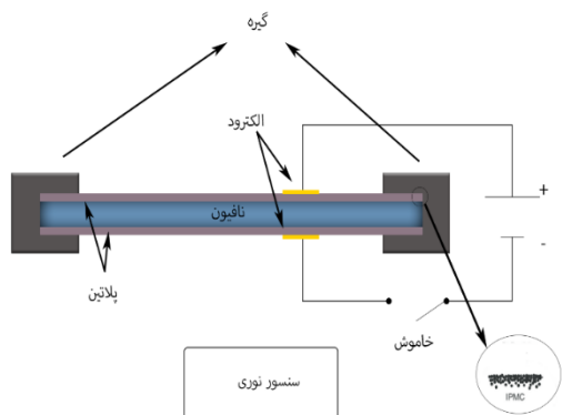
شکل ۵) شماتیک تیری از جنس کامپوزیت پلیمر یونی- فلزی تحت ولتاژ گذرا
