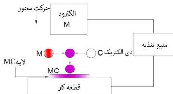
شکل ۱) شماتیک فرایند پوشش دهی تخلیه الکتریکی [3]
