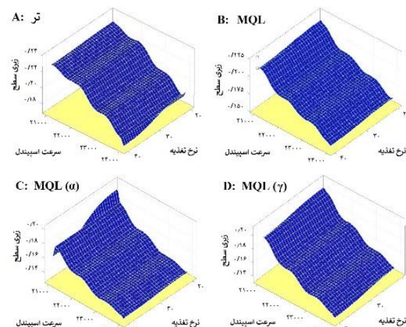
شکل ۸ تاثیر همزمان دو پارامتر سرعت اسپیندل و نرخ تغذیه برای حالت‌های مختلف روانکاری با پایه روغن گیاهی. (A روانکاری تر ، B) روانکاری با روانکار بدون نانوذره به روش MQL، (C) روانکاری با روانکار حامل نانوذره اکسید آلومینیوم آلفا به روش MQL و (D) روانکاری با روانکار حامل نانوذره اکسید آلومینیوم گاما به روش MQL
