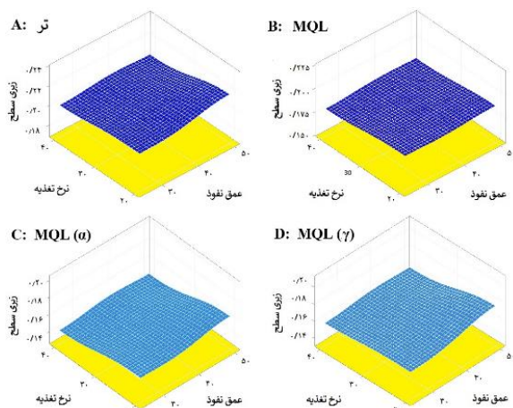
شکل ۷ تاثیر همزمان دو پارامتر نرخ تغذیه و عمق نفوذ برای حالت‌های مختلف روانکاری با پایه روغن گیاهی. (A روانکاری تر ، B) روانکاری با روانکار بدون نانوذره به روش MQL، (C) روانکاری با روانکار حامل نانوذره اکسید آلومینیوم آلفا به روش MQL و (D) روانکاری با روانکار حامل نانوذره اکسید آلومینیوم گاما به روش MQL
