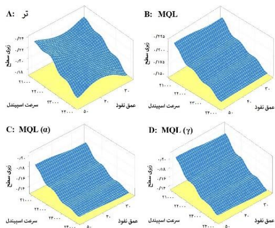
شکل ۶ تاثیر همزمان دو پارامتر سرعت اسپیندل و عمق نفوذ برای حالت‌های مختلف روانکاری با پایه روغن گیاهی. (A روانکاری تر ، B) روانکاری با روانکار بدون نانوذره به روش MQL، (C) روانکاری با روانکار حامل نانوذره اکسید آلومینیوم آلفا به روش MQL و (D) روانکاری با روانکار حامل نانوذره اکسید آلومینیوم گاما به روش MQL
