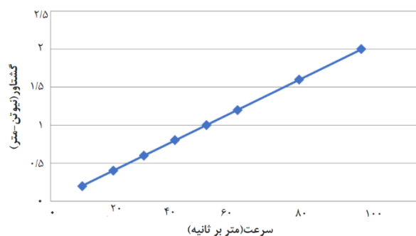
شکل ۸) نمودار تغییرات گشتاور دورانی برحسب تغییرات سرعت جریان هوای تونل باد برای مدل استوانه ۳ باله‌ای
