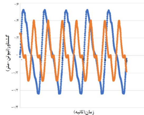
شکل ۶) نمودار نتایج عددی تغییرات گشتاور برحسب زمان برای دوران مدل استوانه ۲ باله ای به مدت ۵ ثانیه
