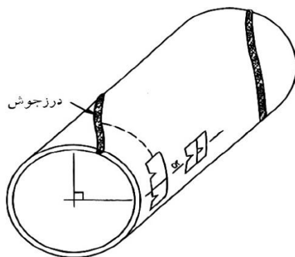
شکل ۲) موقعیت استخراج نمونه‌های استاندارد شارپی از لوله API X70 با درز جوش مارپیچ [22]
