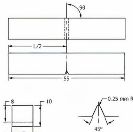
شکل ۱) اندازه نمونه‌ی استاندارد شارپی مورد استفاده در این تحقیق [21]
