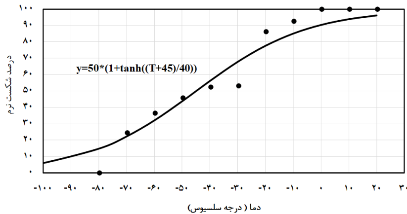
شکل ۵) نمودار درصد شکست نرم نمونه‌های شاپی بر حسب دما و برازش نمودار تانژانت‌هایپربولیک روی داده‌های آزمایشگاهی.
