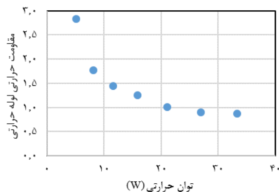
شکل ۸) تغییرات مقاومت حرارتی لوله حرارتی ساخته شده با توان حرارتی
