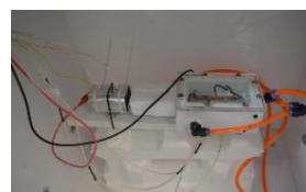
شکل ۴) تجهیزات آزمایشگاهی برای تست مجموعه خنک‌کاری باتری با استفاده از لوله حرارتی
