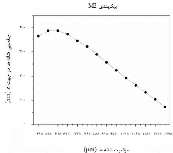
شکل ۵) میزان جابجایی شانه‌ها در اثر اعمال تنش برای پیکربندی M_2
