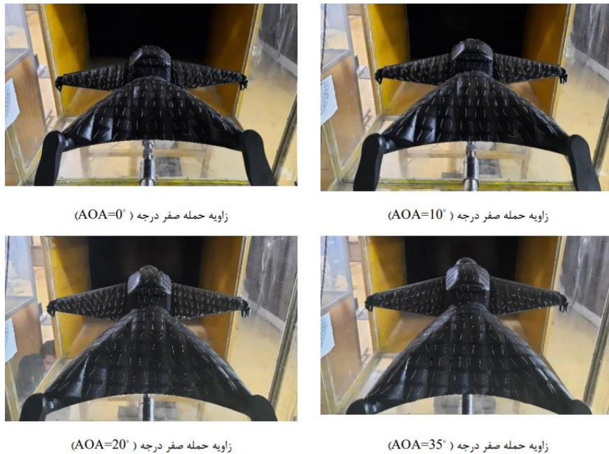
شکل ۹) مریبی سازی جریان روی مدل وینگ سوت در عدد رینولدز 1.5 \times 10^6 در زوایای حمله مختلف
