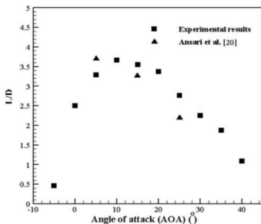
شکل ۱۰) نمودار مقایسه ضریب کارایی وینگ سوت مدل WON7A14 در عدد رینولدز 1.5 \times 10^6
