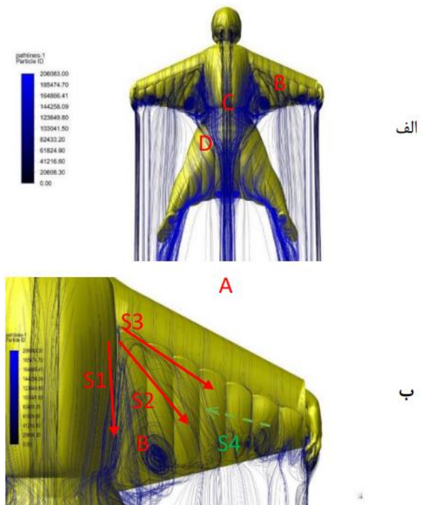
شکل ۱۱) خطوط جریان در زاویه حمله ۱۰ درجه در عدد رینولدز 1/5 \times 10^6 الف: اطراف مدل وینگ سوت ب: روی بال دست HW
