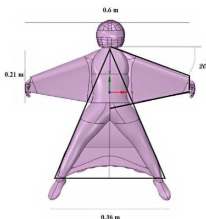
شکل ۲) هندسه و ابعاد مدل وینگ سوت براساس آنتوپومتري بدن صدک ۵۰ ام مرد بالغ
