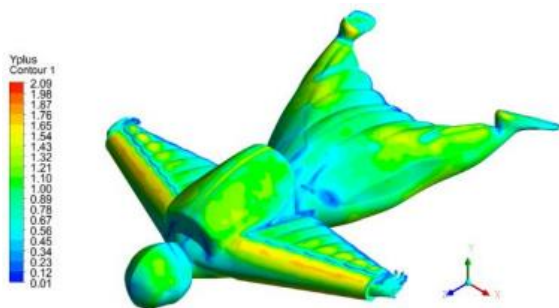
شکل ۷) مقدار y^+ روی مدل مورد مطالعه
