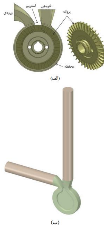
شکل (۱) پمپ بازتولیدکننده؛ (الف) نمای کلی از پمپ بازتولیدکننده [۲۵]، (ب) حجم مفید سیال
