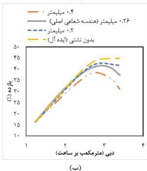
شکل ۱۴) مقایسه پارامترهای عملکردی بر روی انواع مختلف پروانه با لقی‌های جریان متنوع: (الف) نمودار اختلاف فشار، (ب) نمودار بازده
