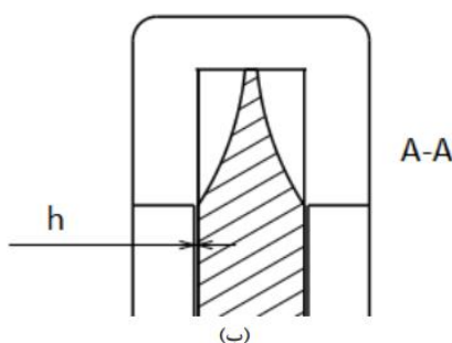
شکل (۲) نمایش جانمایی متغیر هندسی h برای پمپ بازتولیدکننده
