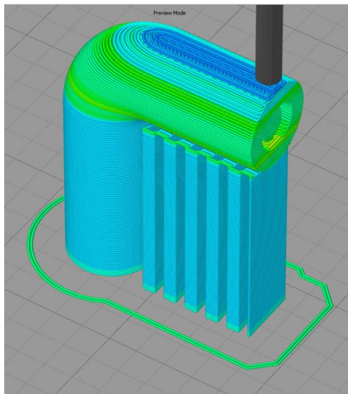
شکل ۱) ساختار تکیه‌گاه که باعث کاهش کیفیت سطح می‌شود
