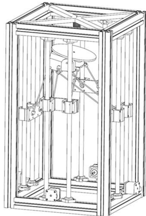
شکل ۲) سازه دستگاه پربینتر سه بعدی ۵ درجه آزادی
