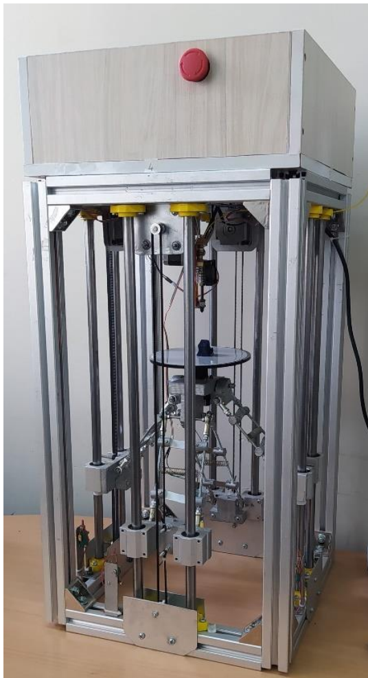
شکل ۴) ربات پربینتر پنج درجه آزادی با مکانیزم موازی
