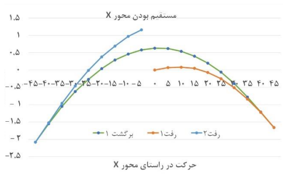
شکل ۱۰ میزان خطای مستقیم بودن حرکت محور X قبل از انجام تنظیمات
