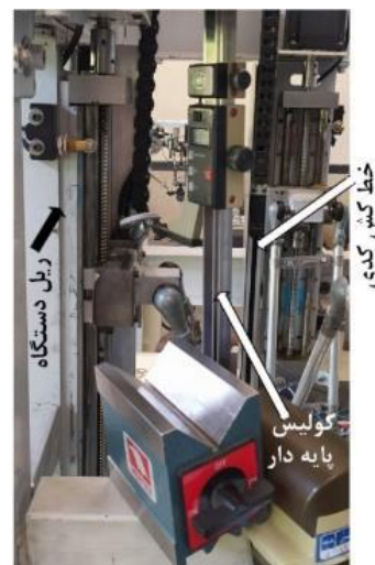
شکل ۶) اندازه‌گیری خطاهای موقعیت‌دهی محورهای حرکتی
