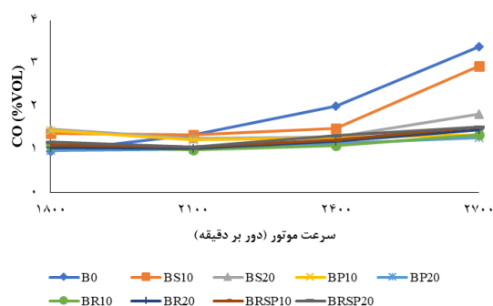
شکل ۱۰) تغییرات آلایند CO موتور با سرعت‌های مختلف برای سوخت‌های آزمایش شده
