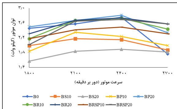
شکل ۴) تغییرات توان موتور در سرعت‌های مختلف برای سوخت‌های آزمایش شده
