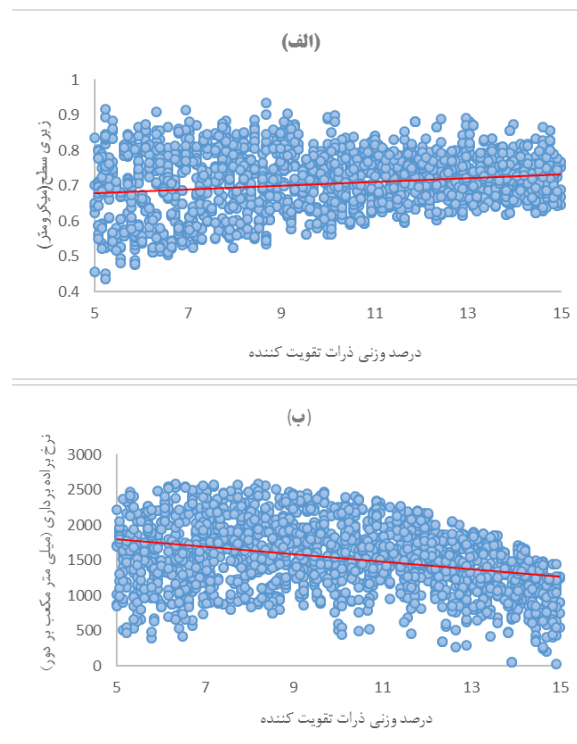
شکل ۱۰) نمودار چگونگی رفتار درصد ذرات تقویت کننده الف) بر روی رفتار زبری سطح ب) بر روی رفتار نرخ براده برداری
