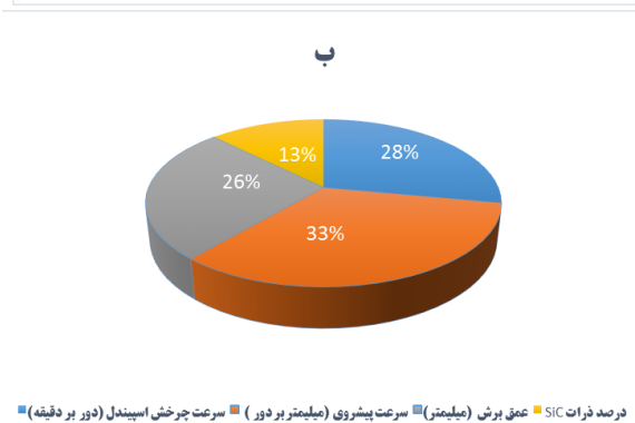
شکل ۹) نمودار درصد تأثیر پارامترهای فرآیند الف) بر روی رفتار زبری سطح ب) بر روی رفتار نرخ براده برداری
