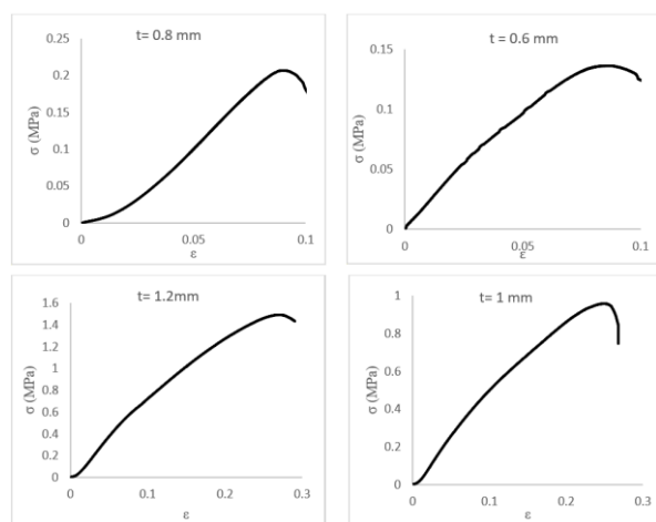
شکل ۵) گراف فشار شبه الاستاتیکی توسط تست فشار برای چهار نمونه سلول آگزیتک با ضخامت های ۰/۶، ۰/۸، ۱ و ۱/۲ میلی‌متر
