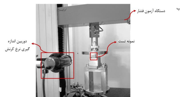
شکل ۴ (الف) سلول های آگزیتک متخلخل ساخته شده به روش DLP، (ب) دستگاه آزمون فشار
