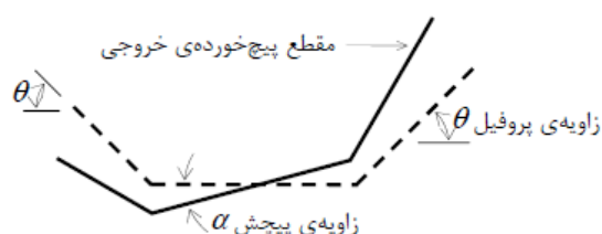
شکل (۱) مقطع پیچ خورده کانال
