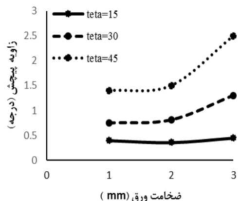
شکل ۷) بررسی اثر ضخامت ورق بر زاویه پیچش با قطر سوراخ ۱۵ میلیمتر
