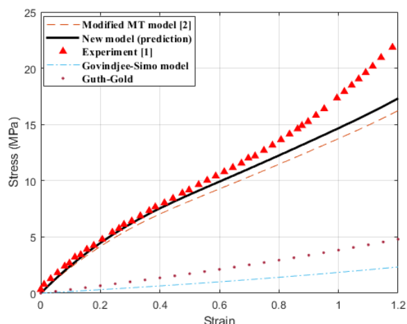
شکل ۳) پیش بینی و مقایسه نتایج رفتار تنش-کرنش در نانوماده مرکب لاستیک طبیعی حاوی ۲۰٪ کربن سیاه با استفاده از مدل تحلیلی خودسازگار بهبود یافته و سایر مدل های مرتبط
