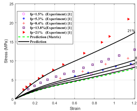
شکل ۴) پیش بینی و مقایسه نتایج رفتار تنش-کرنش در نانوماده مرکب لاستیک طبیعی حاوی درصد های مختلف کربن سیاه با استفاده از مدل تحلیلی خودسازگار بهبود یافته
