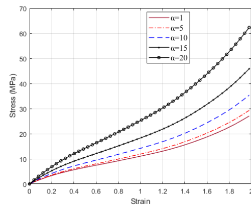
شکل ۵) نتایج رفتار تنش-کرنش در نانوماده مرکب لاستیک طبیعی حاوی کربن سیاه با استفاده از ذرات تقویت کننده با نسبت منطری مختلف و مدل تحلیلی خودسازگار بهبود یافته
