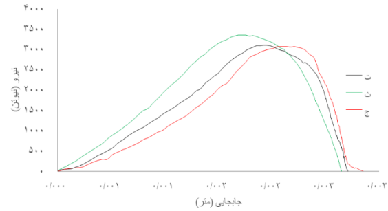
(الف) منحنی نیرو - جایجایی با ارتفاع سقوط ۱۰۰ میلی‌متر شکل ۶) منحنی جایجایی نیرو
