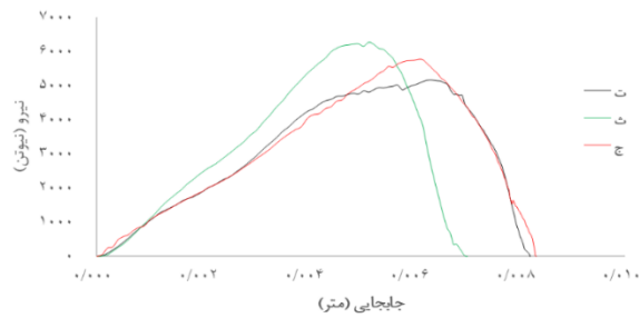
(ب) منحنی نیرو جایجایی به ارتفاع سقوط ۵۰۰ میلی‌متر
