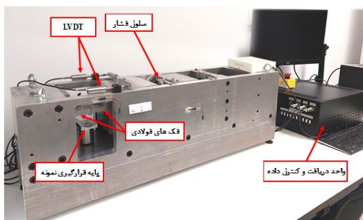
شکل ۲) تجهیزات آزمایش pCT.
