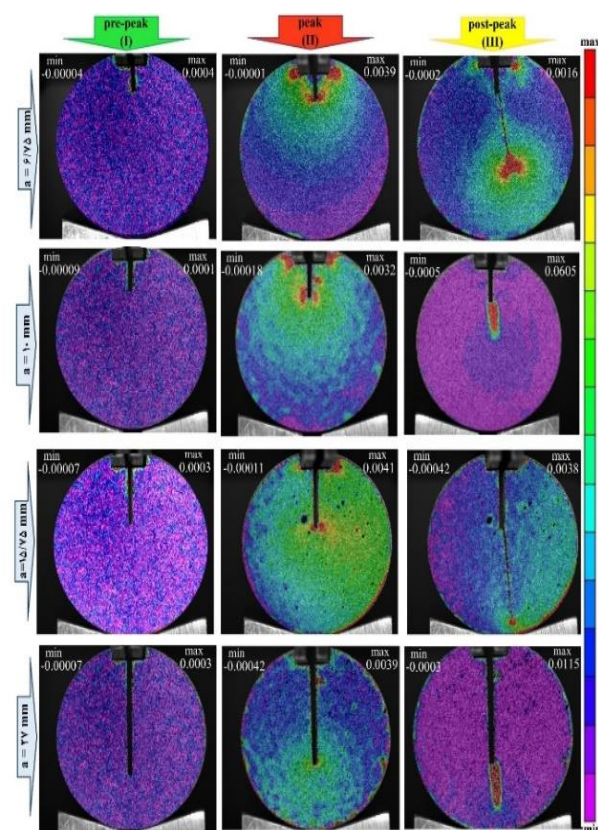
شکل ۹) میدان تغییرشکل حاصل از روش برهم‌نگاری تصاویر دیجیتالی: تصاویر مربوط به وضعیت نمونه در هریک از لحظات پیش (I)، در (II) و پس از (III) بار بیشینه (بترتیب از چپ به راست) و برای طول ترک اولیه ۶/۷۵، ۱۰، ۱۵/۷۵ و ۲۷ میلی‌متر (بترتیب از بالا به پایین).
