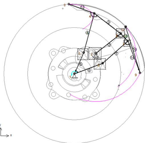
شکل ۵ تغییر موقعیت مفاصل در حالت کاملاً باز در محیط نرم افزار SAM
