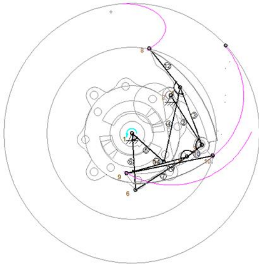
شکل ۶ تغییر موقعیت مفاصل در حالت کاملاً بسته در محیط نرم افزار SAM
