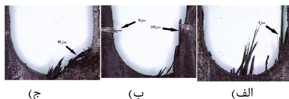
شکل ۳) انواع لایه لایه شدگی
