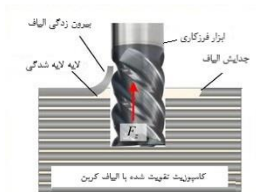
شکل (۲) نحوه برش صفحه کامپوزیتی
