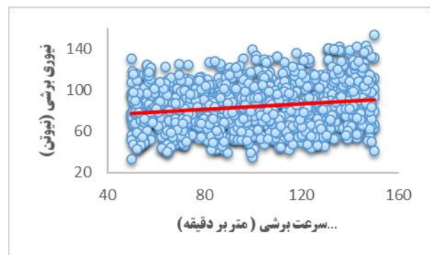
شکل ۴ اثر سرعت برشی بر زبری نیروهای ماشین کاری
