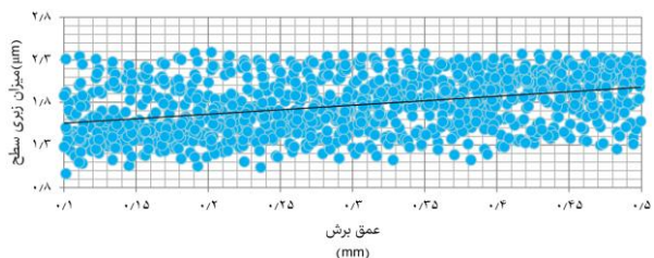
شکل ۶) نمودار تغییرات زبری سطح با افزایش عمق برش
