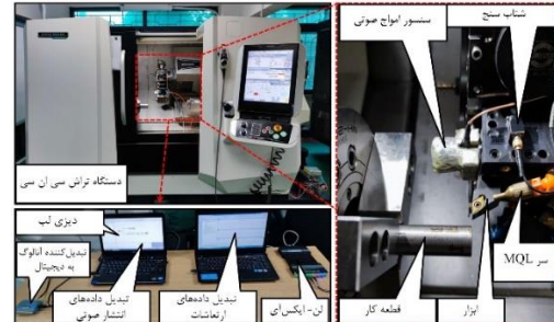
شکل (۱) تجهیزات انجام آزمایش [۱۸]
