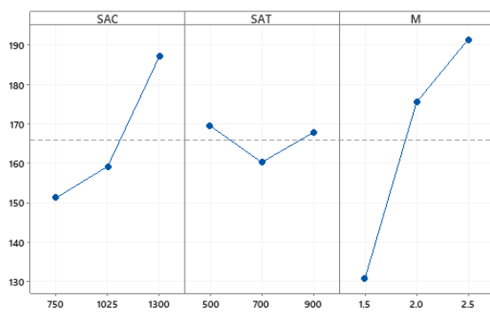
شکل ۱) نمودار اثر پارامترهای مورد بررسی بر زمان ماشین‌کاری
