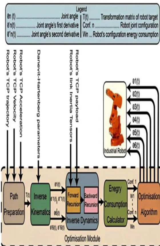
شکل ۶. نمونه ای از به حداقل رساندن مصرف انرژی برای حرکت بازوی ربات [۱۳].
