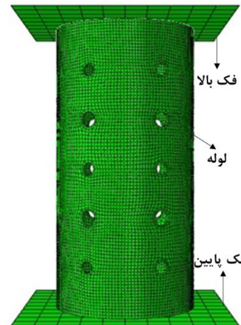
شکل (۲) مدل المان محدود استفاده شده
