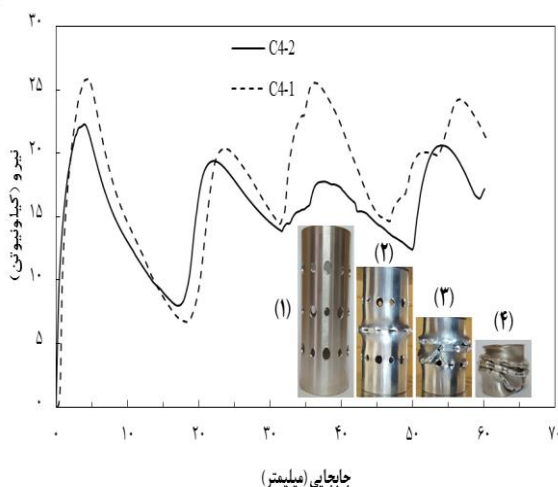
شکل ۱۰) نمودار نیرو-جابجایی آزمایش C4
