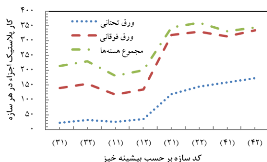
نمودار ۶) کار پلاستیک اجزاء - بیشینه خیز عددی در هر سازه
