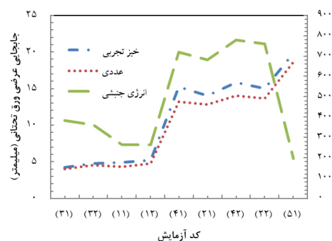
نمودار ۷) خیز ورق تحتانی بر حسب انرژی جنبشی کل در هر سازه
