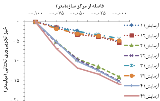
نمودار ۴) خیز ورق تختانی بر حسب فاصله از مرکز سازه به روش عددی
