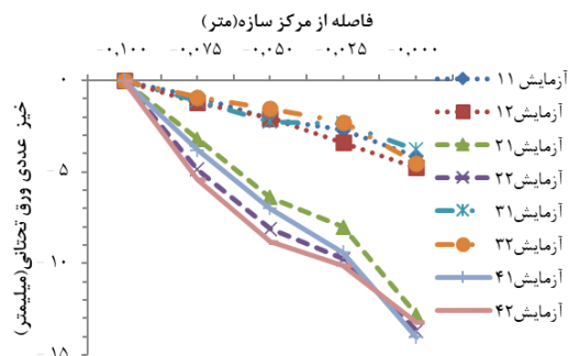
نمودار ۳) خیز ورق تختانی بر حسب فاصله از مرکز سازه به روش عددی
