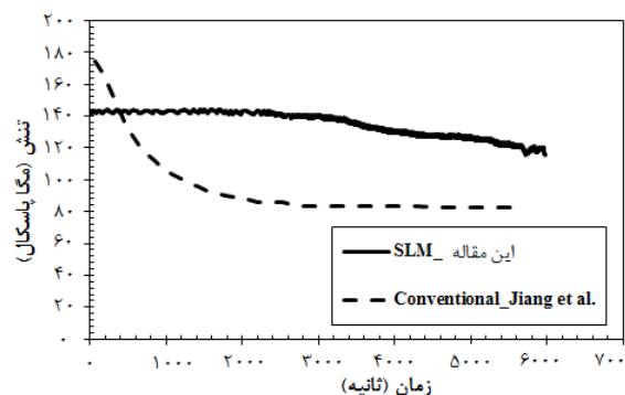
شکل ۸) نمودار تجربی رهایش تنش سوپر آلیاژ (IN718) ساخته شده به روش (SLM) و مرسوم [21] در دمای ۶۵۰ درجه سانتیگراد
