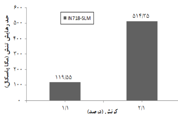
شکل ۷) نمودار حد رهایش تنش سوپر آلیاژ (IN718) ساخته شده به روش (SLM)، تحت دمای آزمایش ۶۵۰ درجه سانتیگراد و کرنش‌های ۱۲/۱٪ و ۲۲/۱٪
