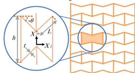
شکل ۱) نمایی از سازه آگزتیک میکروسلولی و سلول واحد آن
