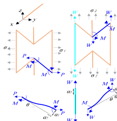
شکل ۲) پاسخ میکروسلول آگزتیک تحت بارگذاری کششی
