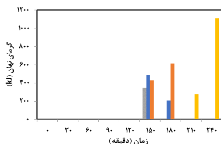
شکل ۸) تغییر در مقدار گرمای نهان برای مقادیر مختلف پارافین با گذشت زمان
