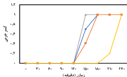
شکل ۷) تغییر کسر جرمی پارافین با زمان
