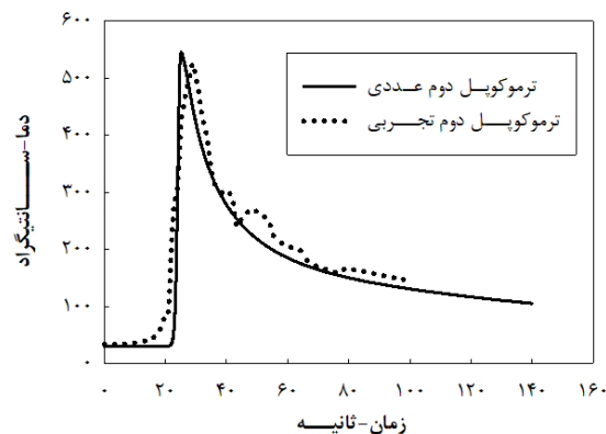
شکل ۴) مقایسه توزیع دما در محل ترموکوپل دوم
