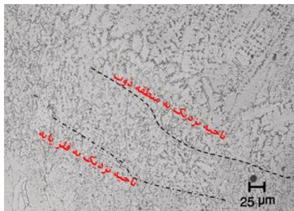
شکل ۷) تصویر میکروسکوپ نوری از ناحیه متأثر از حرارت
