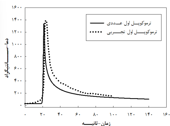
شکل ۳) مقایسه توزیع دما در محل ترموکوپل اول
