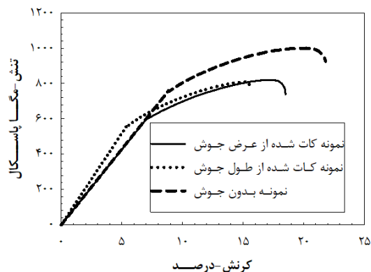
شکل ۱۰) نمودار تنش-کرنش نمونه جوشکاری نشده، نمونه تهیه شده از عرض جوش و نمونه تهیه شده از طول جوش
