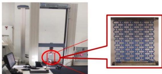
شکل (۶) دستگاه تست کشش مدل
