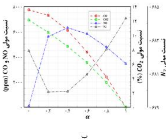
شکل ۱۰ (الف) رادیکال‌ها، (ب) گونه‌ها نسبت‌های مولی بدست آمده در شرایط درصد آمونیاک متفاوت: (الف) رادیکال‌ها، (ب) گونه‌ها
