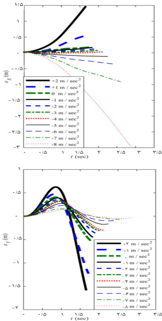
شکل ۶) خطای تعقیب موقعیت طولی و موقعیت عرضی کنترل یکپارچه برای سناریو اول
