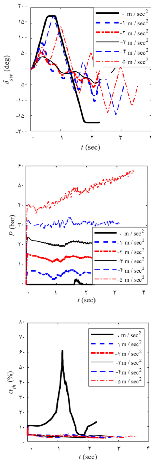
شکل ۹) ورودی‌های کنترلی کنترل سناریو دوم
