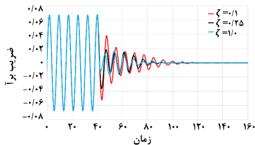
شکل ۱۳) تغییرات ضریب برای استوانه در سه حالت \zeta=0.1 ، \zeta=0.25 و \zeta=1.0 به ازای r=2 ، A=0.01 و f=0.1 - شروع کنترل از زمان t=40 (محورها بدون بعد)
