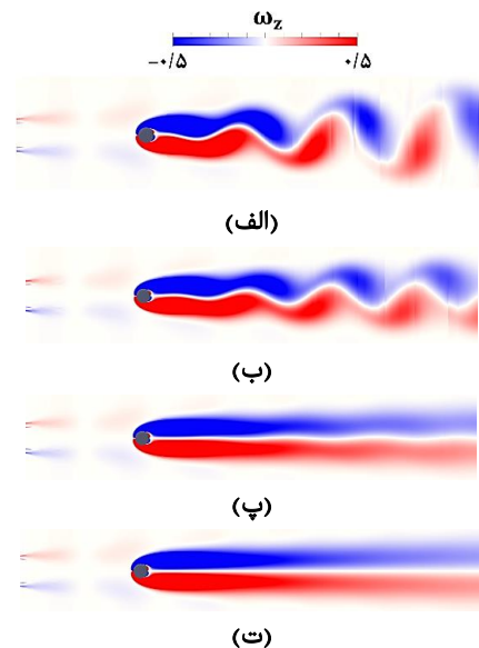
شکل ۱۰) کانتور ورتیسیتهی لحظه‌ای جریان روی استوانه حاوی اغتشاش ورودی (۱۹) با شرایط A=0.05 ، f=0.1 ، Re=0.1 و r=2 در فواصل زمانی \Delta t=40 با شروع از زمان اعمال کنترل
