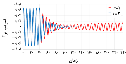
شکل ۱۱) تغییرات ضریب برای استوانه در دو حالت r=1 و r=2 به ازای A=0.01 ، \zeta=0.1 و f=0.1 - شروع کنترل از زمان t=40 (محورها بدون بعد)
