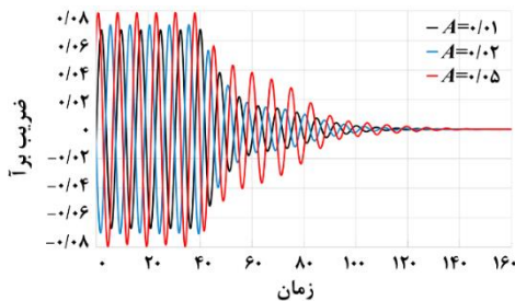
شکل ۱۲) تغییرات ضریب برای استوانه در سه حالت A=0.01 ، A=0.02 و A=0.05 به ازای r=2 ، \zeta=0.1 و f=0.1 - شروع کنترل از زمان t=40 (محورها بدون بعد)
