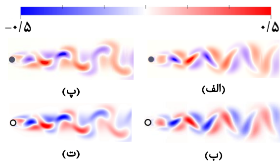
شکل ۵) کانتور ورتیسیتهی موده‌های OTD دوران‌یافته در حالت ناپایای سیکل محدود استوانه. الف و ب) مود اول OTD، پ و ت) مود دوم OTD. الف و پ) نتایج پژوهش حاضر. ب و ت) تصاویر مستقیم مرجع [9].
