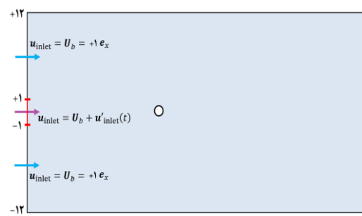
شکل ۹) اعمال ورودی اغتشاشی پریودیک متغیر با زمان در مرز سیستم
