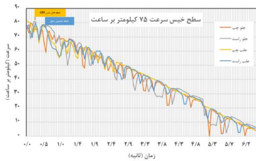
شکل ۵) سرعت ۷۵ کیلومتر بر ساعت در سطح خیسی، چرخ جلو سمت چپ
