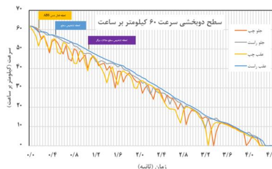
شکل ۱۰) تفاوت زمانی تشخیص سطح الگوریتم پیشنهاد شده در دو مقاله فوق و این پژوهش در چرخ جلو سمت چپ در سرعت ۶۰ کیلومتر بر ساعت بر روی سطح دوبخشی
