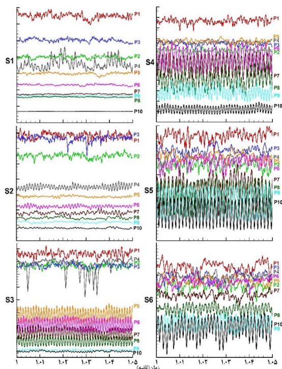
شکل ۶) تغییرات نسبت فشار انتهای لوله در فاصله‌های مختلف بین نازل و لوله
