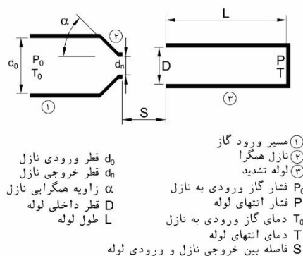
شکل ۲) طرحواره لوله تشدید هارتمن اسپرنگر
