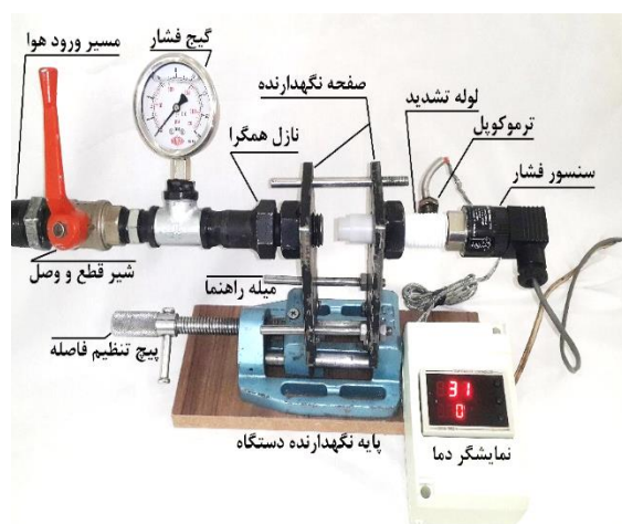
شکل (۵) تصویر میز آزمایش
