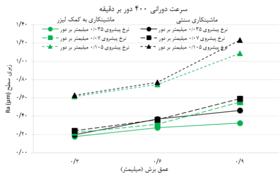
شکل ۶ مقایسه تاثیر مقادیر متفاوت نرخ پیشروی و عمق برش بر کیفیت زبری سطح قطعه کار در تراشکاری سنتی و تراشکاری به کمک لیزر
