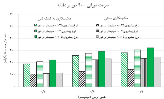
شکل ۵) مقایسه تأثیر مقادیر مختلف نرخ پیشروی و عمق برش بر دمای براده در تراشکاری سنتی و تراشکاری به کمک لیزر
