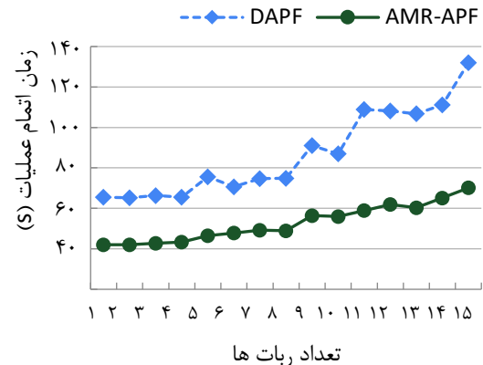
شکل ۱۲) مقایسه زمان اتمام عملیات در شبیه‌سازی عملیات طراحی مسیر جمعی در نقشه یکسان و با تعداد ۱ تا ۱۵ ربات.
