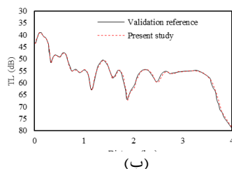
شکل ۳) (الف) هندسه محیط انتشار صدا برای اعتبارسنجی کد عددی [12] و (ب) نمودار افت تراپدی برای گیرنده در عمق ۳۰ متری؛ با استفاده از نرم افزار for3d در مقایسه با پژوهش مرجع اعتبارسنجی.
