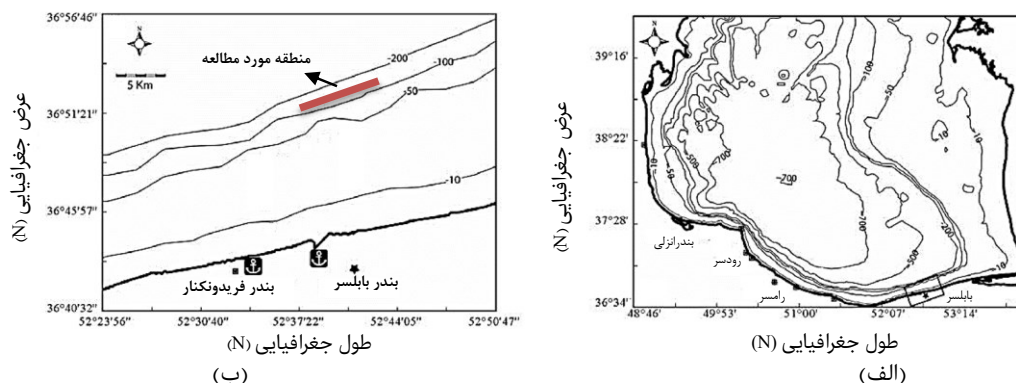
شکل ۱) (الف) منطقه جنوب دریای خزر، (ب) محل منطقه مورد مطالعه در این تحقیق.
