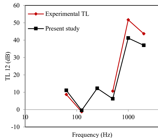
شکل ۴) اعتبارسنجی شبیه‌سازی با داده تجربی؛ مقایسه افت تراپردی بین نقطه ۱ و ۲ در دو حالت داده تجربی و شبیه‌سازی.
