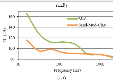
شکل ۹) (الف) تغییر ضریب تنکشی بستر و (ب) اثر آن بر افت تراوردی.
