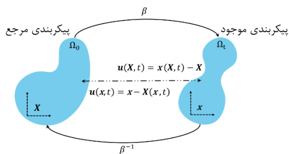
شکل ۴) توصیف نگاشت بین پیکربندی‌های اولیه و فعلی.
