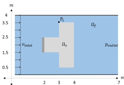
شکل ۱۰ هندسه و شرایط مرزی مسئله دوم
