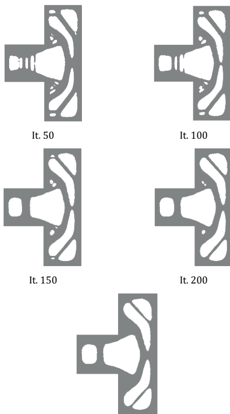
شکل ۱۳ تکامل توپولوژی بهینه برای زمان t = 0.032 ثانیه
