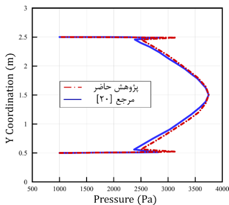
شکل ۷) فشار وارد بر مرز سمت چپ سازه در پژوهش حاضر و مرجع [20]
