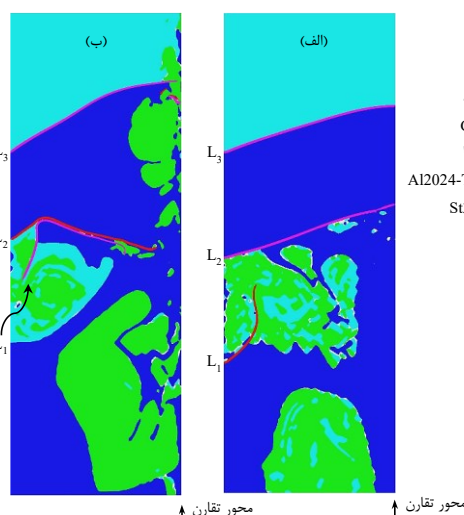
شکل ۸) پاسخ ساختارهای نوعی با C_1^{med} هوا، C_2^{med} آب و لایه میانی AI2024-T3 و (ب) St37
