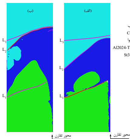
شکل ۹) پاسخ ساختارهای نوعی با C_1^{med} آب، C_2^{med} هوا و لایه میانی AI2024-T3 و (ب) St37
