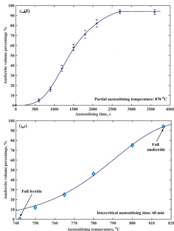
شکل ۵) تغییرات درصد حجمی فاز آسفریت با: (الف) زمان آستنیت‌ه جزئی در دمای ۸۷۰ °C، (ب) دمای آستنیت‌ه بین بحرانی به مدت ۶۰ دقیقه.
