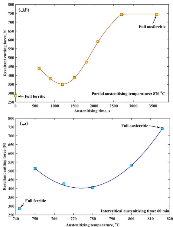
شکل ۶) تغییرات نیروی برش برآیند با: الف) زمان آستنیت‌دهی جزئی در دمای ۸۷۰ °C، ب) دمای آستنیت‌دهی بین بحرانی به مدت ۶۰ دقیقه.
