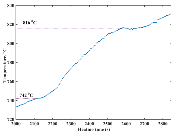
شکل ۲) نمایش نحوه تغییر دمای مرکز نمونه چدن نشکن در یک کوره مقاوم‌تی در بازه زمانی ۳۰ تا ۵۰ دقیقه بعد از شروع گرمایش .
