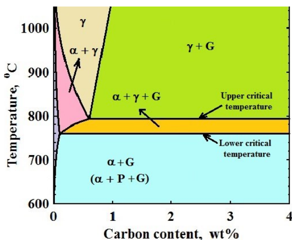
شکل (۱) برش هم ترکیب نمودار فاز \text{Fe-C-Si} تائی سه تائی \text{Fe-C-Si} ، مقطع 2/4 درصد وزنی سیلیسیم [۸] .
