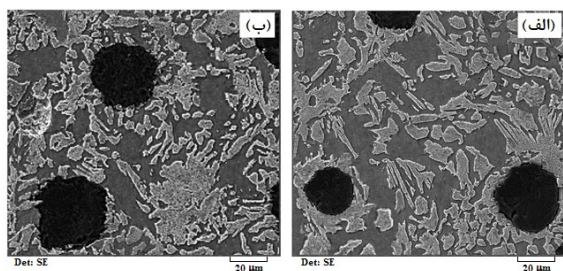
شکل ۴) تصاویر میکروسکپ الکترونی روبشی از ریزساختار نمونه‌های دوفازی فریتی-آسفریتی تولید شده با فرایند: (الف) آستنیت‌ه جزئی در دمای ۸۷۰ °C به مدت ۲۰ دقیقه، (ب) آستنیت‌ه بین بحرانی در دمای ۸۷۰ °C به مدت ۶۰ دقیقه.
