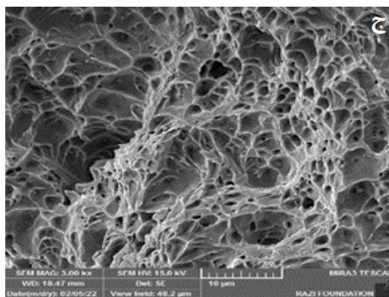
شکل ۵) تصاویر SEM از مقطع شکست نمونه ضربه فلز جوش E7018 در دمای محیط (الف) مورفولوژی دیمپلی سطح شکست (ب) حفرات و دیمپل‌ها در ساختار (ج) حفرات و دیمپل‌ها در نمای نزدیک‌تر
